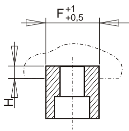
SECCION A-A SECTION A-A
