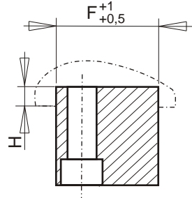
SECCION B-B SECTION B-B
